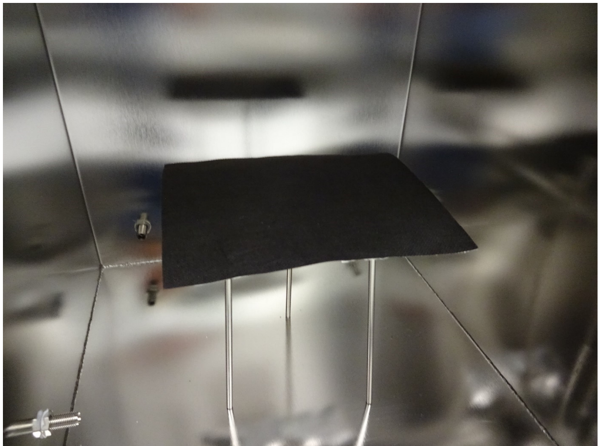
Abbildung 1: Probe „btf EASY WALL AL NEW“ in der Prüfkammer
